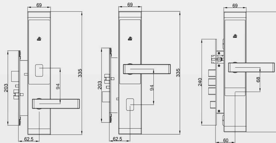
标配7B锁体
