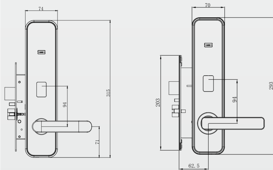
标配7B锁体
