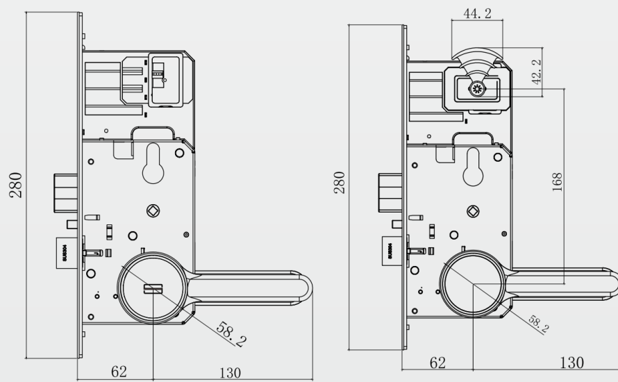
标配11A锁体
