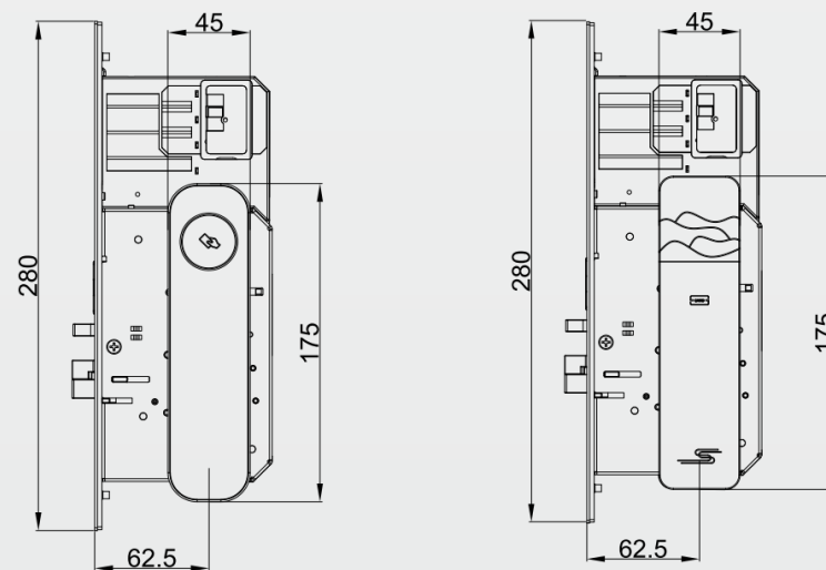
标配12A锁体
