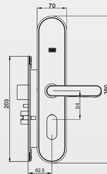
标配7B锁体
