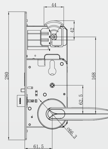
标配11A锁体
