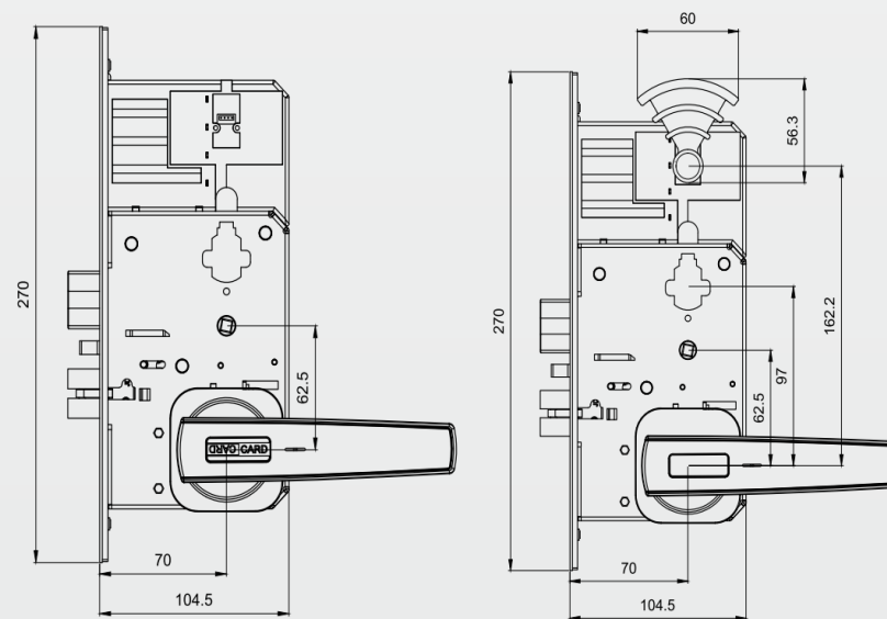
标配6B号锁体
